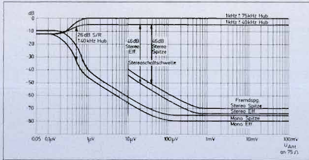
FM-Fremdspannungsabstand in Abhängigkeit von der Antennenspannung
