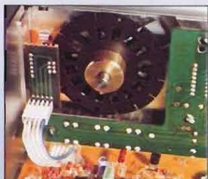
Handabstimmung mit magnetisch rastendem Drehknopf und Optokoppler
